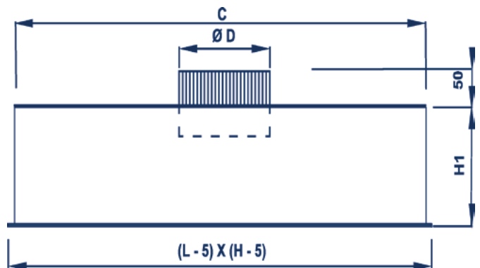
SFT 786T+ PL/V (plenum vertical)
